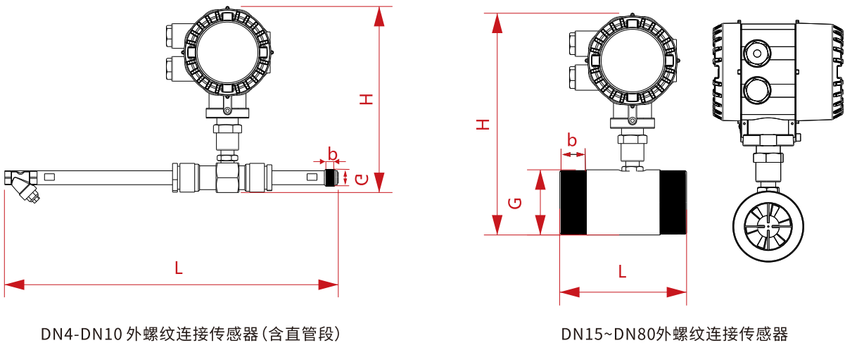
图7-1 外螺纹连接示意图
