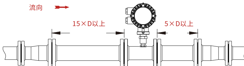
图8-2 扩管安装示意图
