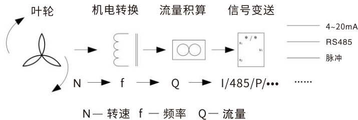
图3-1 工作原理图
