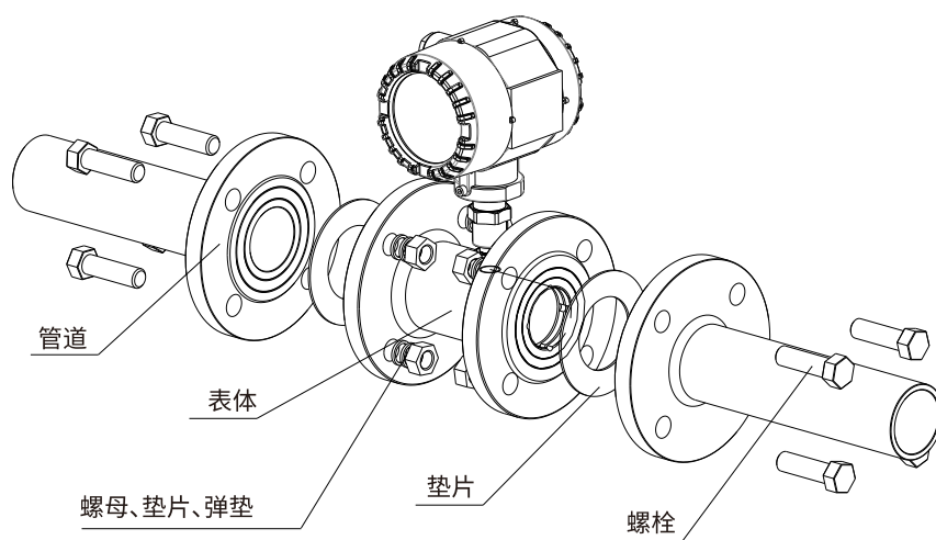
图8-7 法兰对接型示意图
