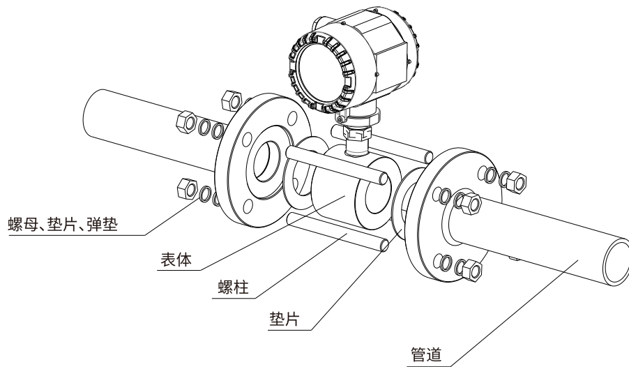
图8-9 法兰夹持型示意图
