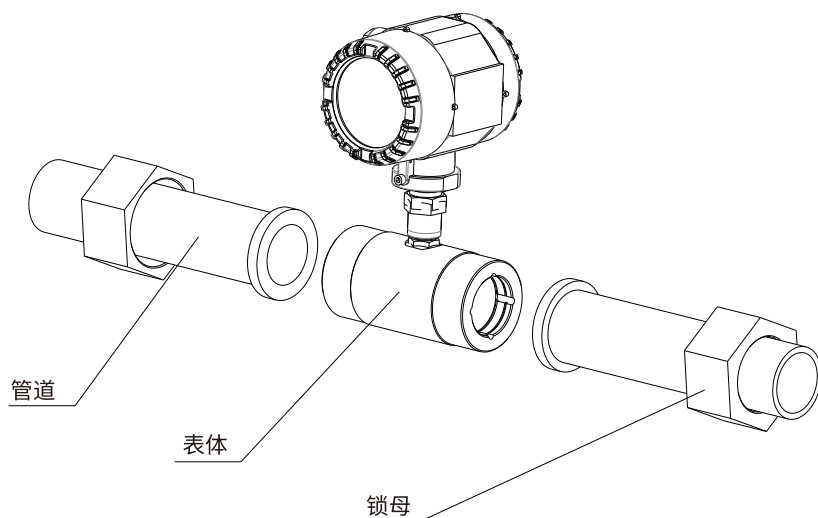
图8-8 螺纹连接型示意图
